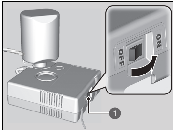
❶ Công Tắc Bơm Nén Khí
