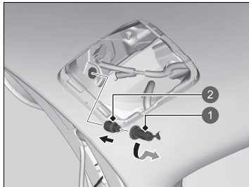
❶ Đui
