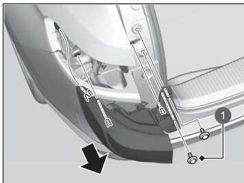
① Bu-lông
