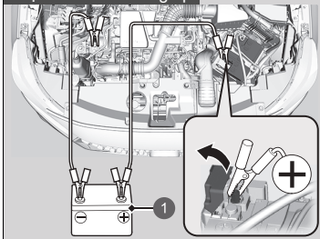
1 Ắc Quy Hỗ Trợ
