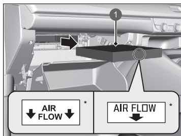
❶ Lọc Gió Điều Hoà
