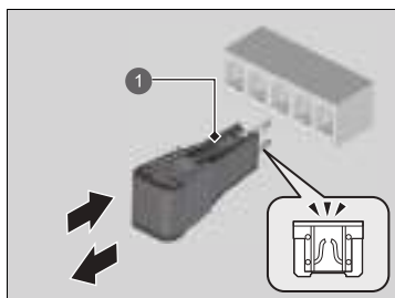
❶ Kẹp Cầu Chì
