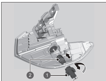
① Đui ② Bóng Đèn
